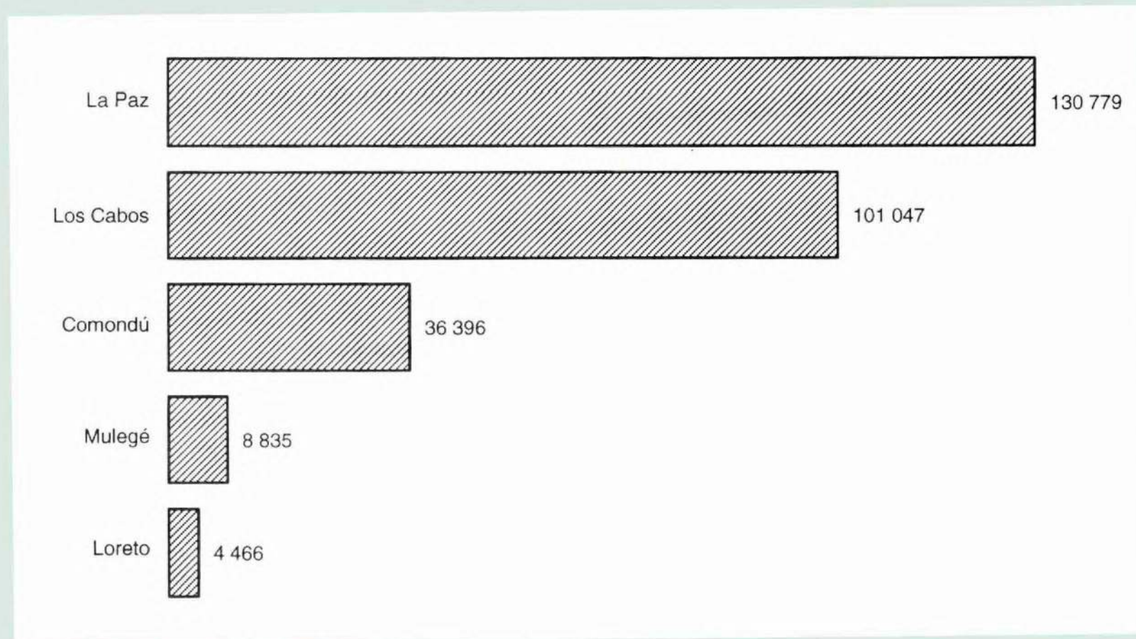
Automóviles registrados en circulación por municipio Al 31 de diciembre de 2008
